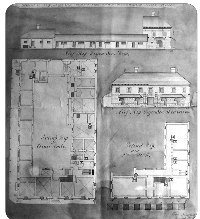
A szegedi városháza tervrajza 1799-ből.
